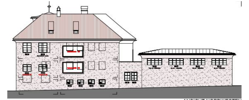
ANSICHT NORDWESTEN
