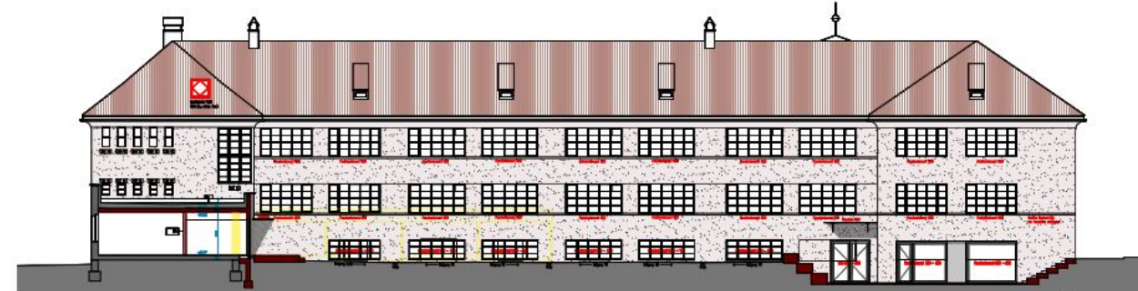
ANSICHT SÜDWESTEN
